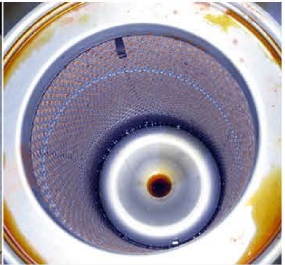
Mobil SHC Rarus 46으로 9,500시간 가동 후 육안검사 시 비교적 깨끗한 외관을 유지
